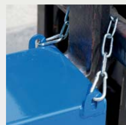
Bezpečnostní pojistky.
